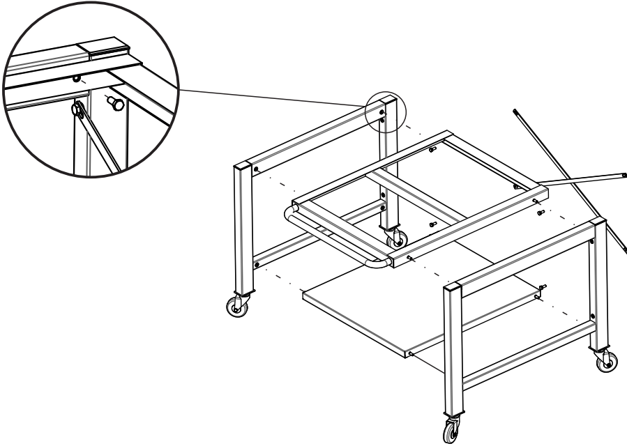
Fig 1 : Coloque los laterales sobre la base y fije los bulones , con sus arandelas correspondientes, a las tuercas remachadas ubicadas en los extremos de la base.
